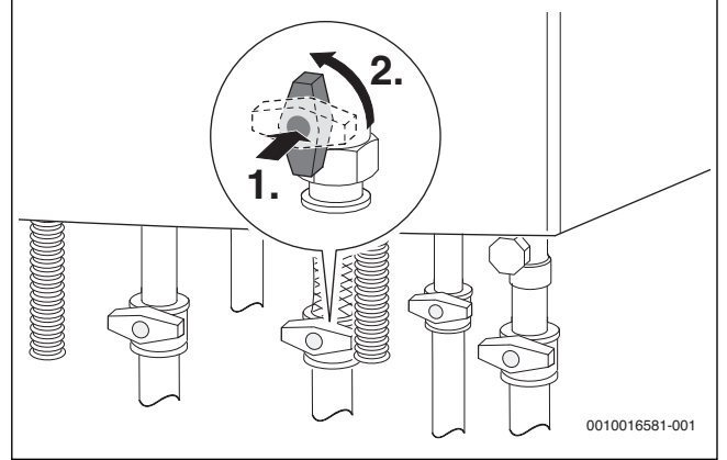
Res. 3 Gaz vanasının açılması
